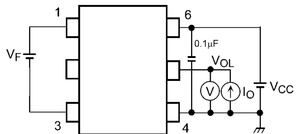
Fig. 13.1.2 IOBL Test Circuit
