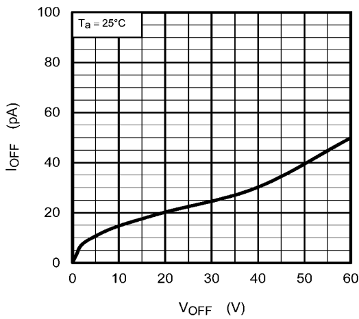
Fig. 13.1.9 I_{OFF} - V_{OFF}
