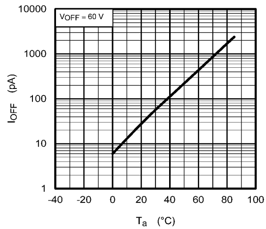
Fig. 13.1.10 I_{OFF} - T_a
