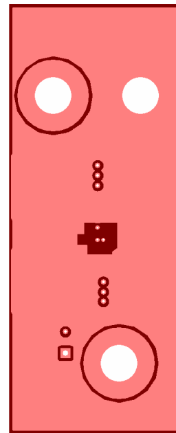
Layer 2 – GND
