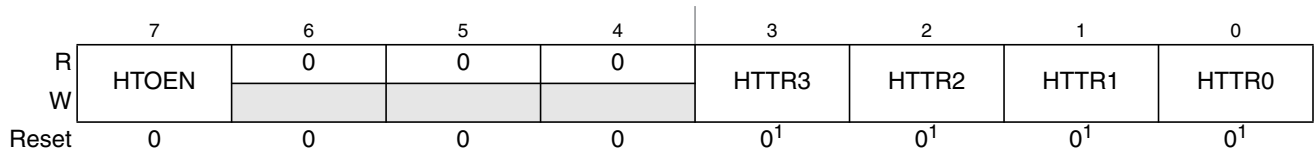
Figure 23-9. VREGHTTR
