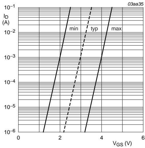
T_j = 25\text{ °C}; V_{DS} = 5\text{ V}
