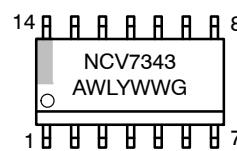
SOIC-14
