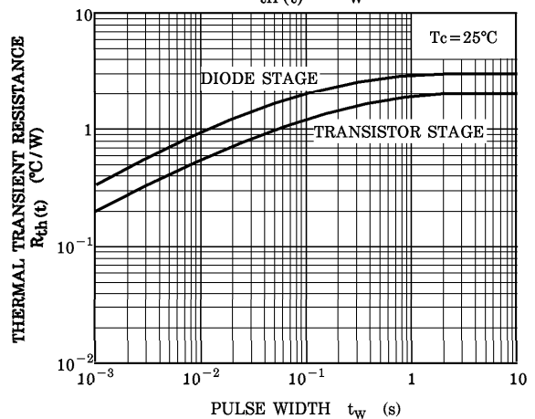
R_{th}(t) - t_w
