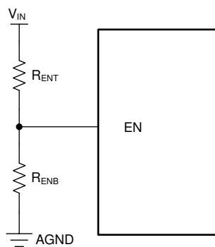
Figure 39. UVLO Using EN
