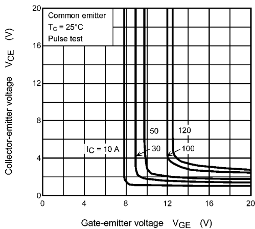
Fig. 8.5 V_{ce} - V_{ge}
