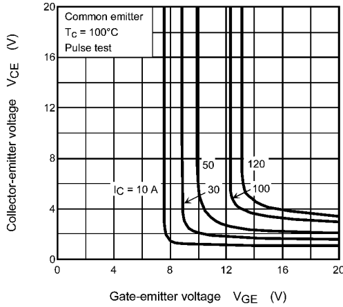
Fig. 8.7 V CE - V GE
