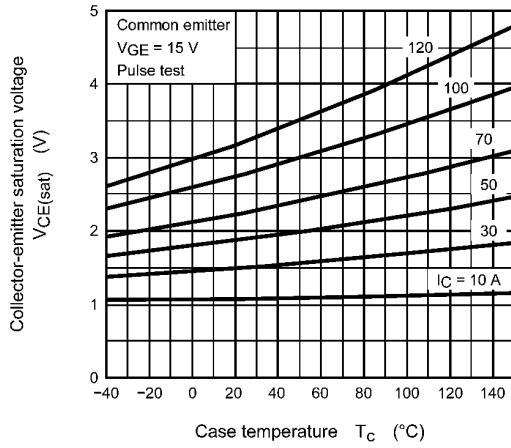
Fig. 8.9 V CE(sat) - T c
