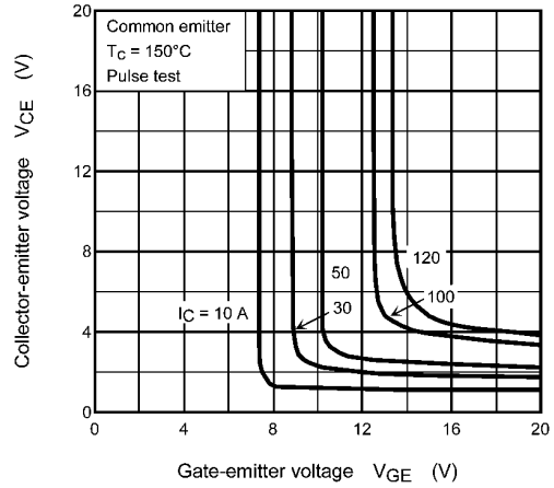
Fig. 8.8 V CE - V GE
