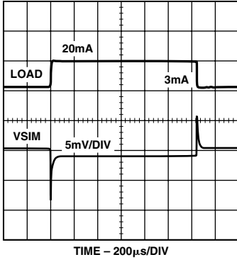
TPC 10. VSIM Load Step
