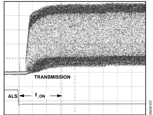
Figure 25. ALS Negate Time, 50 µs/div
