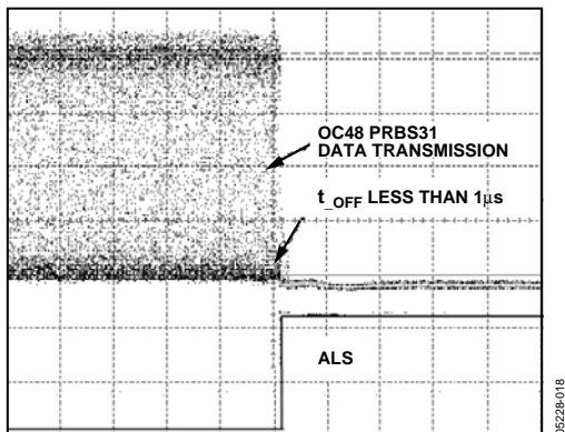
Figure 22. ALS Assert Time, 5 µs/div
