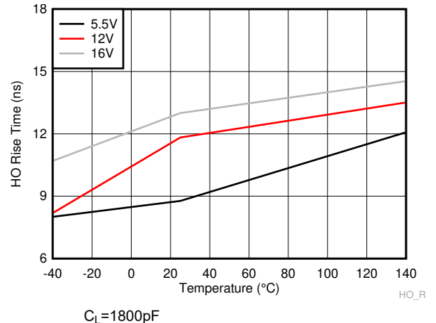
Figure 6-24. HO Rise Time
