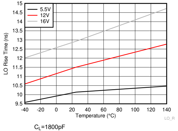
Figure 6-22. LO Rise Time
