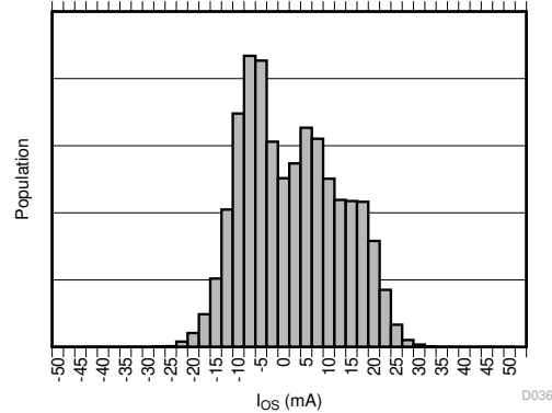
TMCS1101A3U-Q1
