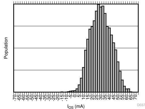
TMCS1101A4U-Q1
