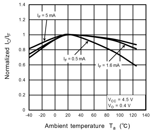
Fig. 12.2.10 I_O/I_F - T_a
