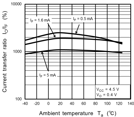
Fig. 12.2.9 I_O/I_F - T_a
