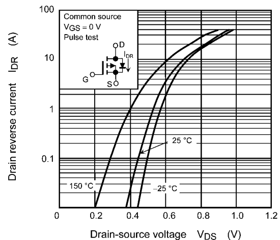
Fig. 8.12 I_{DR} - V_{DS}
