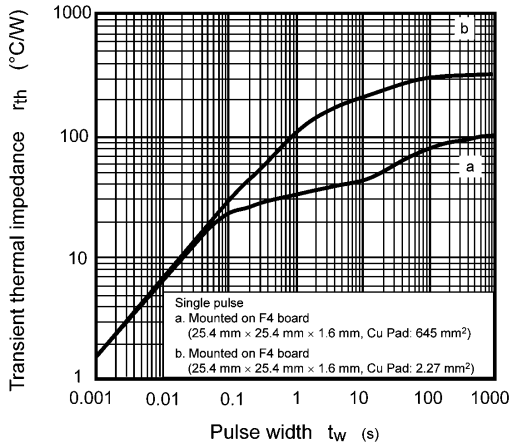
Fig. 8.13 r_{th} - t_w
