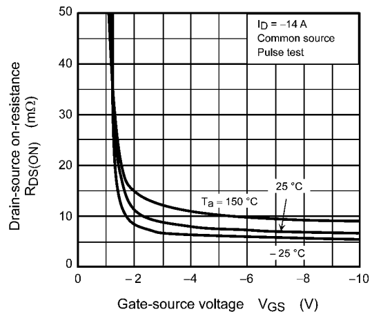
Fig. 8.4 R_{DS(ON)} - V_{GS}
