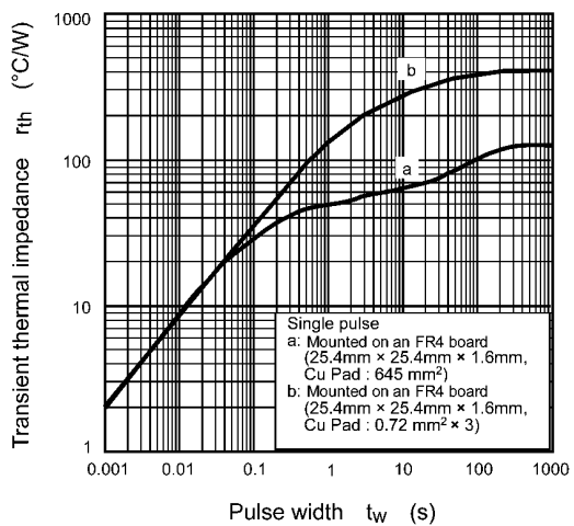
Fig. 8.12 r_{th} - t_w
