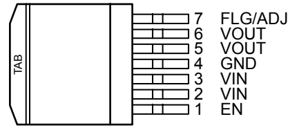
S-PAK-7
