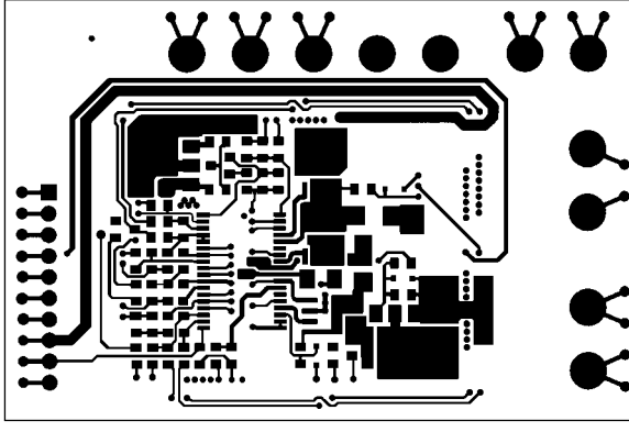
Copper Layer 4
