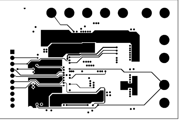
Copper Layer 3
