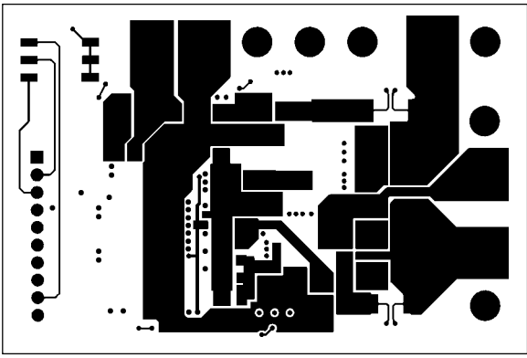
Copper Layer 1
