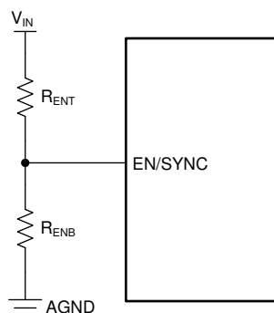
Figure 34. UVLO Using EN
