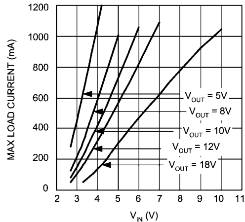
Max. Load Current (typ) vs VIN - "X"
