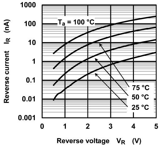
Fig. 7.2 I_R - V_R
