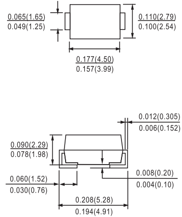
DO-214AC(SMA)
