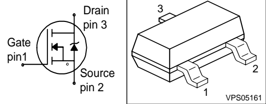
PG-SOT23
