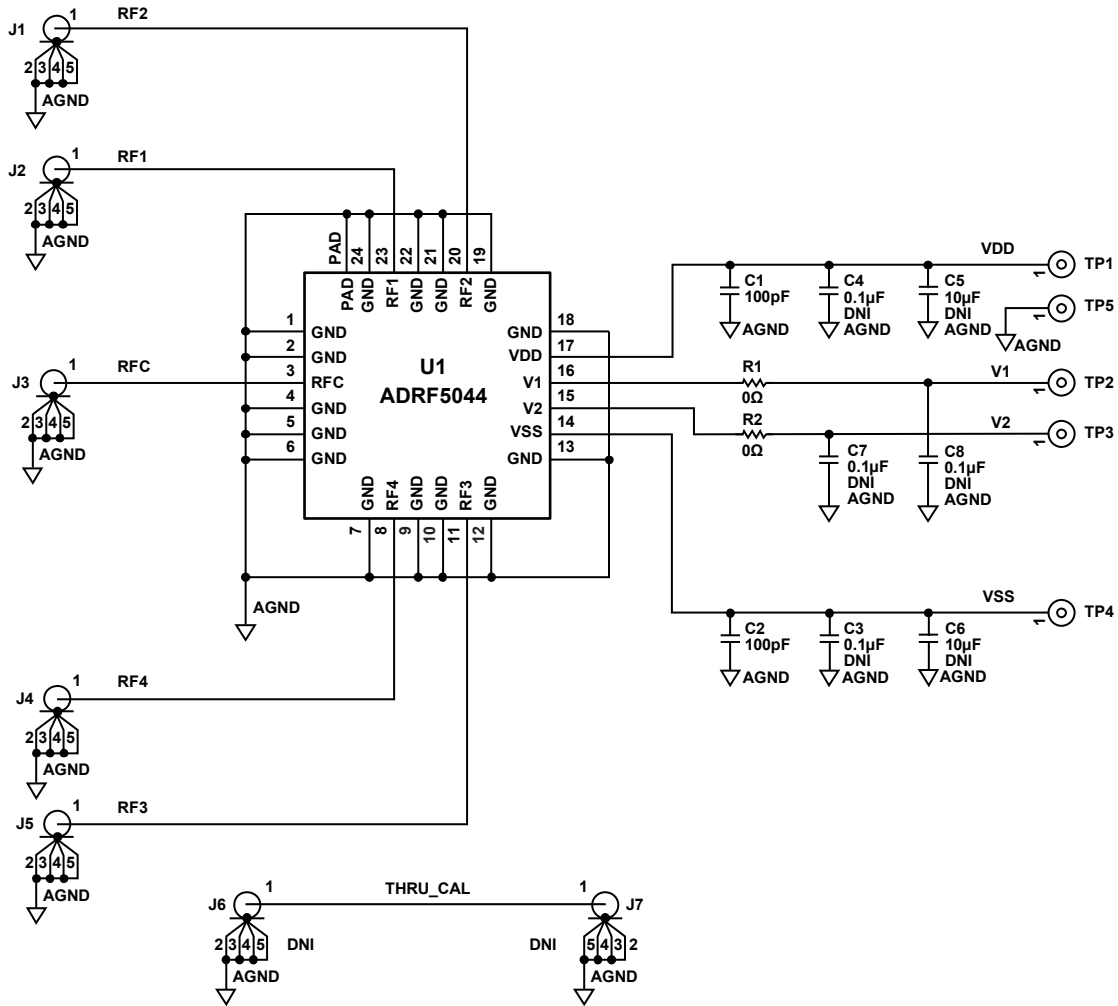
Figure 25. ADRF5044-EVALZ Schematic
