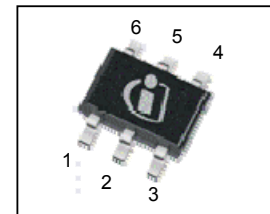
PG-SOT363
