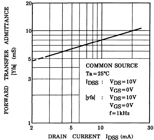
|Y fs | - I DSS
